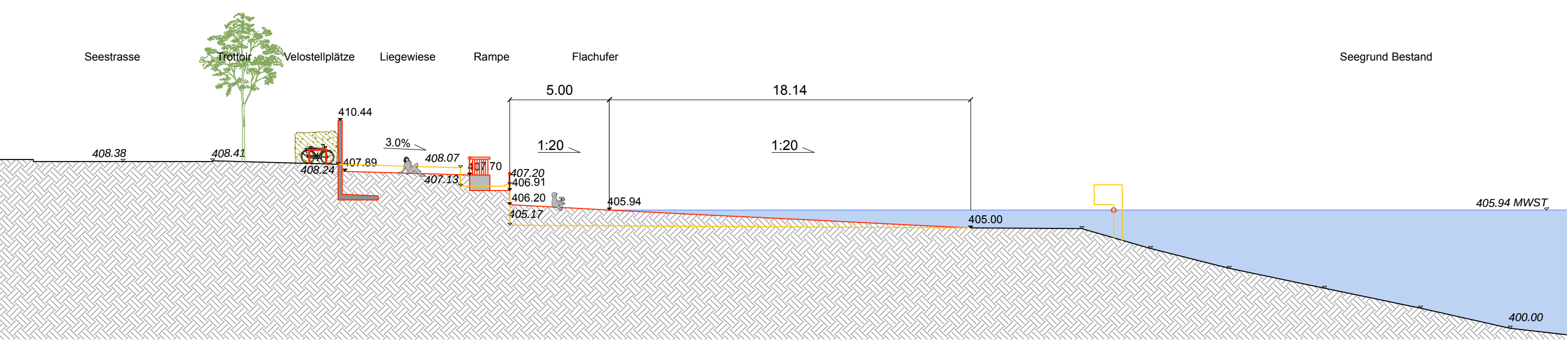
Schnitt 4-4' M 1:200
