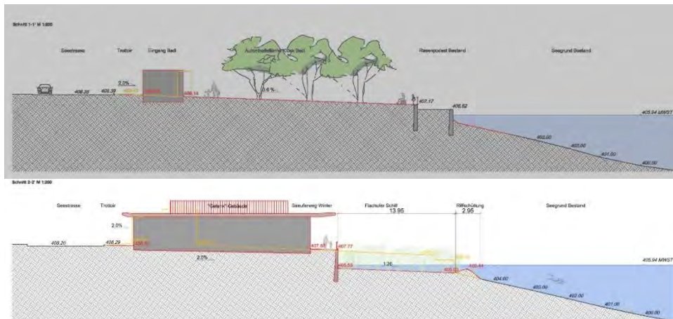
Schnitte durch den Eingangsbereich und das Gelenkgebäude der zusammengeführten Badi, planikum GmbH
