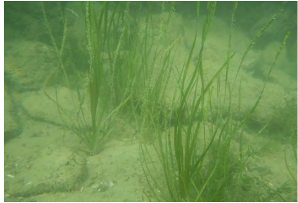
Alisma gramineum im Transekt 11 in 1.2 m Tiefe.
