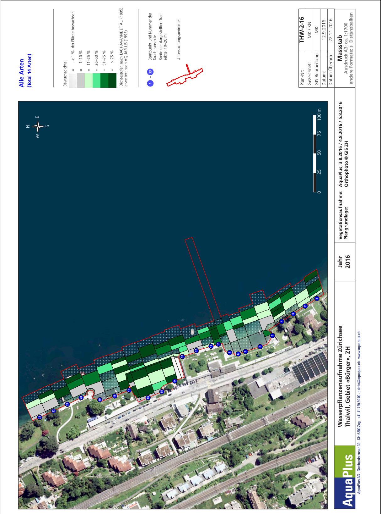
Abb. 12: Plandarstellung der Wasserpflanzen-Gesamtdichte im Untersuchungsperimeter z«Thalwil Bürger». Perimeter = 23 Transekte im Abstand von 10–20 im Bereich «Bürger», Zürichsee, Thalwil, Kanton ZH. Vegetationsaufnahme: 3.8.2016 / 4.8.2016 / 5.8.2016. Für weitere Betrachtungen (Artverbreitung, Untergrundbeschaffenheit etc.) siehe PLANDARSTELLUNGEN.
