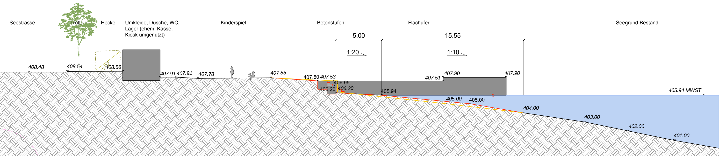
Schnitt 6-6' M 1:200
