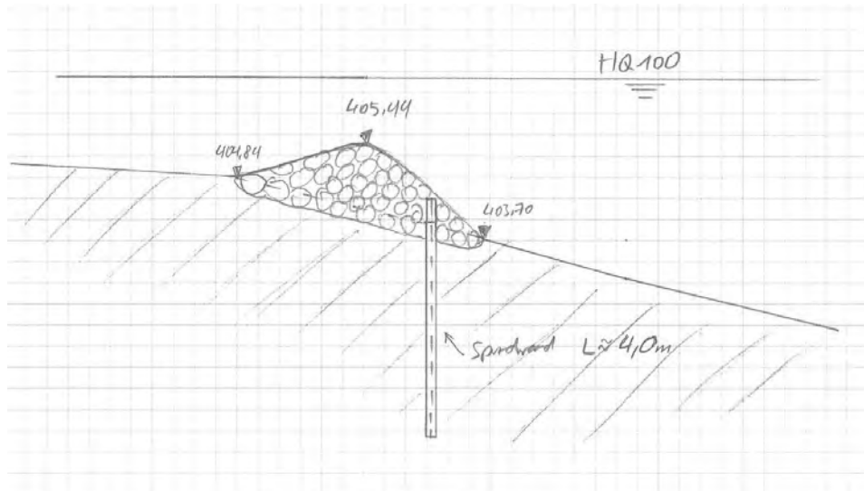
Skizze Spundwand zur Stabilisierung der Riffschüttung, IG Sihl-Entlastungsstollen
