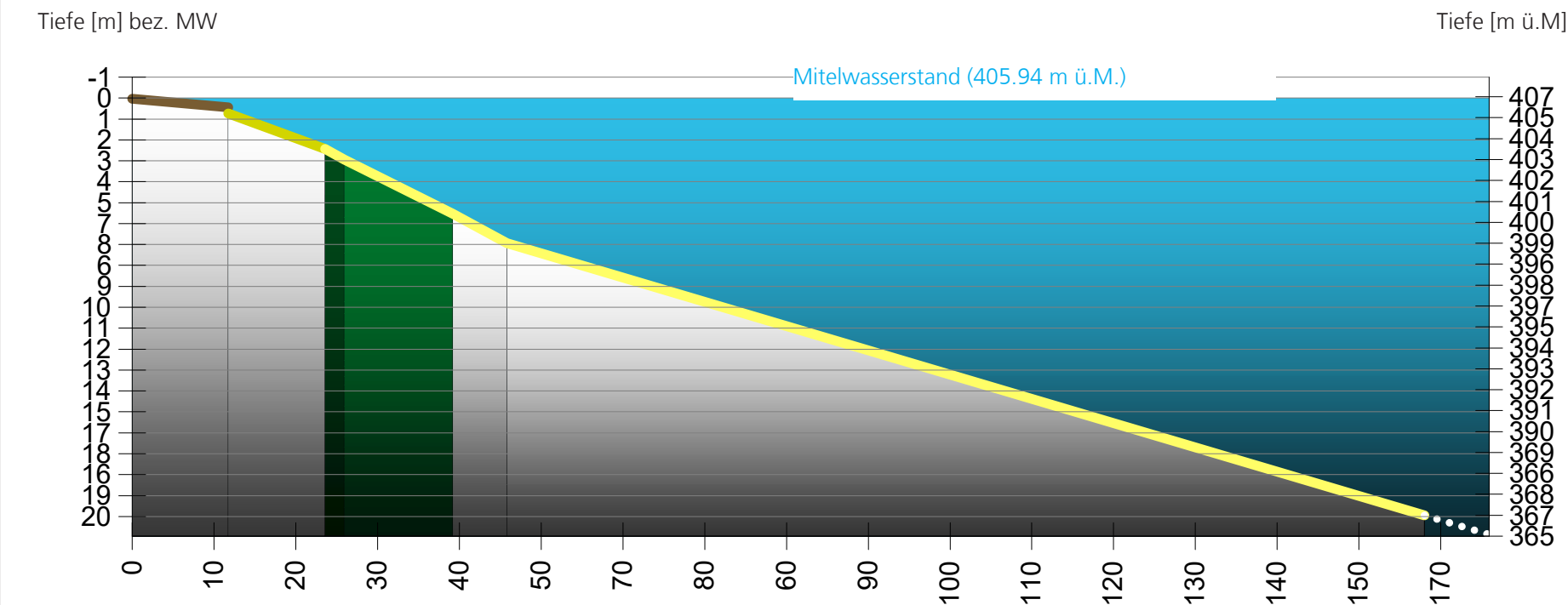
Transekt 9 – ganze Länge
