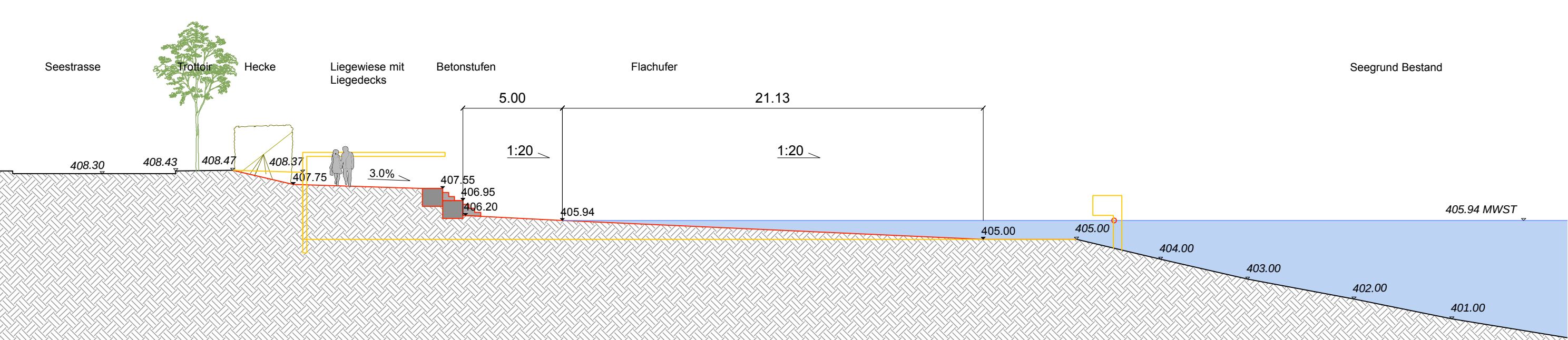
Schnitt 5-5' M 1:200
